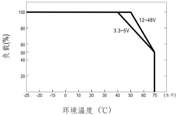
■ 减额曲线
